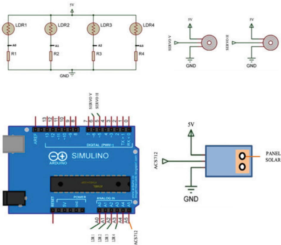
Figura 2 Diseño del prototipo de un sistema de control y seguimiento mediante servomotores
