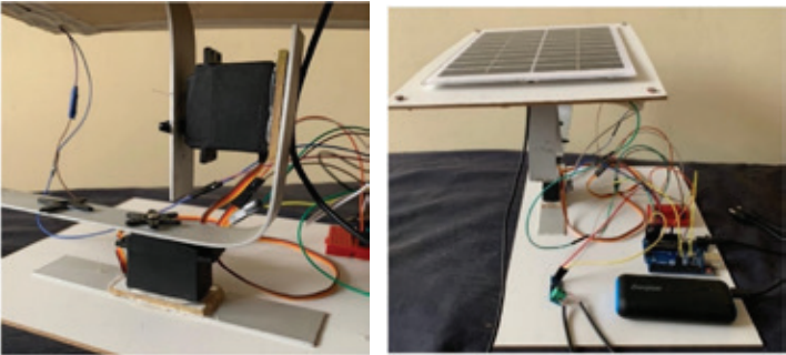
Figura 2 Diseño del prototipo de un sistema de control y seguimiento mediante servomotores
