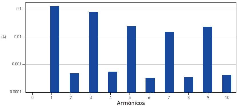
Figura 9 Armónicos de corriente
