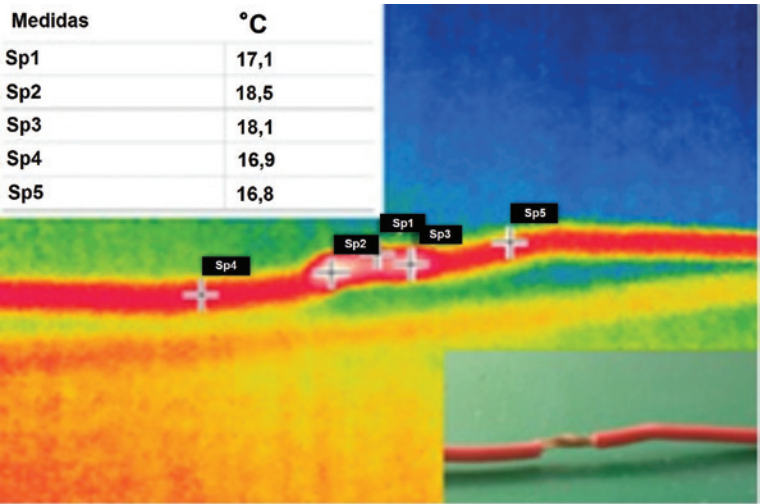
Figura 11 Temperatura del conductor neutro
