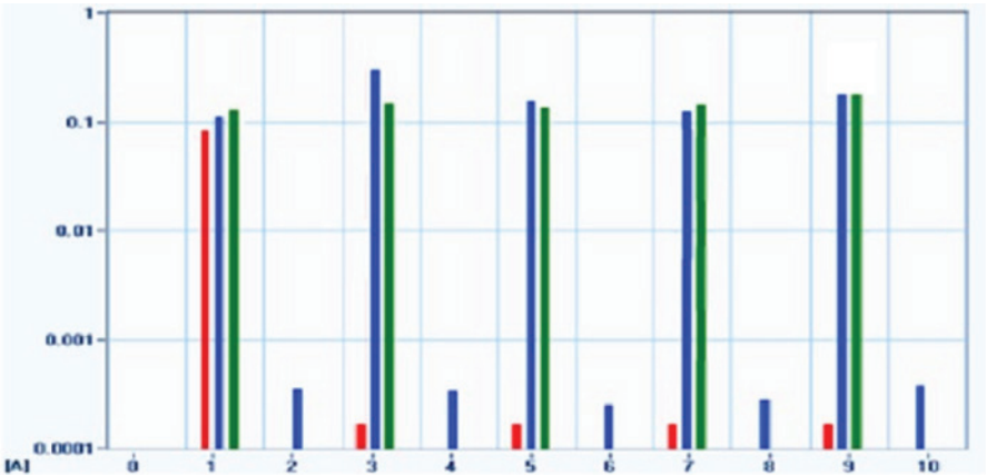
Figura 10 Armónicos de corriente
