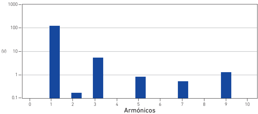
Figura 8 Armónicos de tensión
