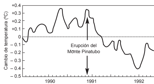
Figura 4 Erupción del monte Pinatubo en Filipinas, en 1991, y su efecto en la temperatura global.
