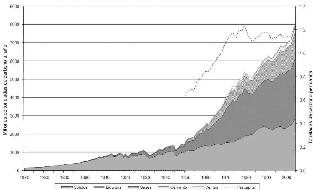
Figura 6 Emisiones de carbono antropogénicas desde 1870 (1 t C = 3,66 t CO 2 )
