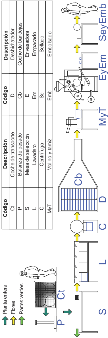
Figura 6. Esquema del proceso productivo de flores de manzanilla común en bolsas filtrantes Elaboración propia
