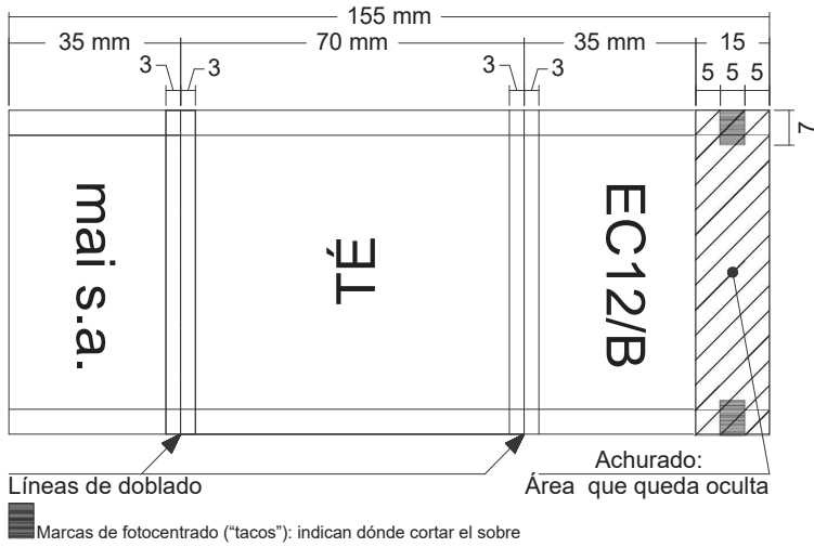
Figura 14. Medida estándar de sobre de envoltura abierto para envasadora Maisa EC12/B
