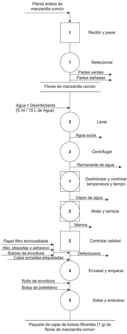
Figura 8. Diagrama de operaciones de proceso Elaboración propia
