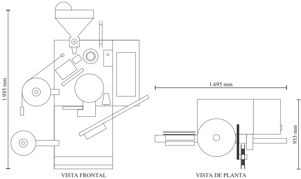
Figura 15. Dimensiones de envasadora argentina modelo Maisa EC12/B
