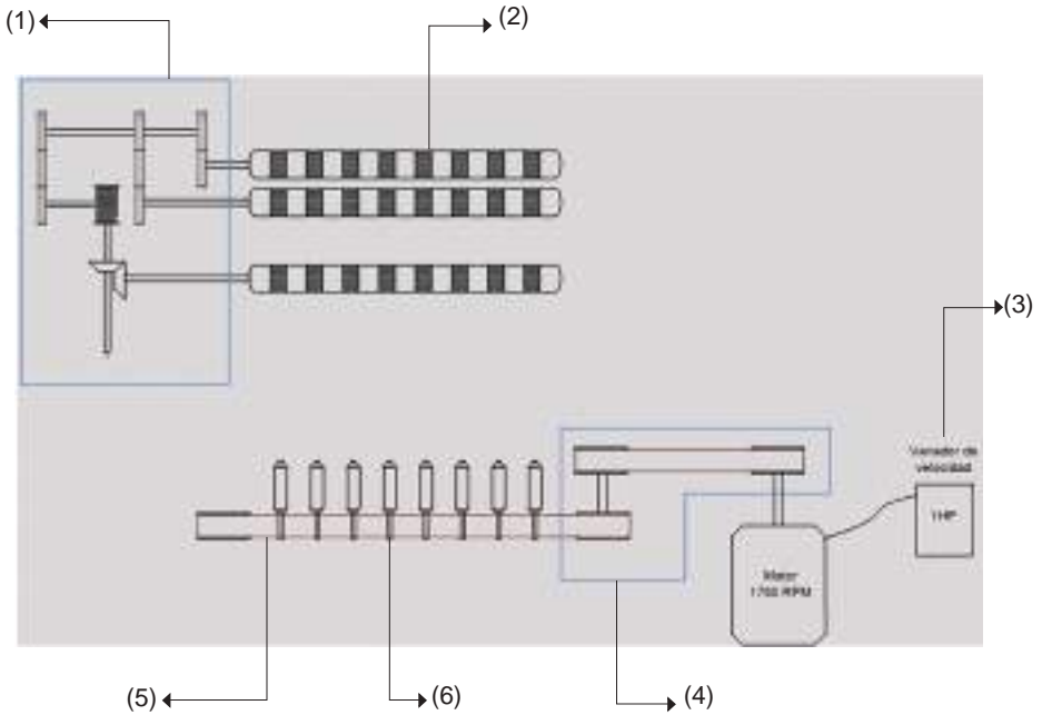
Figura 4. Cadena cinemática que brinda velocidad a los husos y al tren de estiraje Elaboración propia
